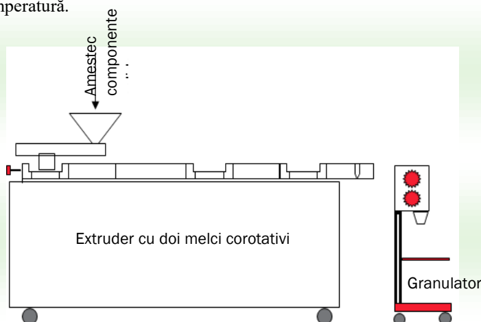
Fig. 1 - Instalația de realizare a fertilizanților granulari pe bază de lână
